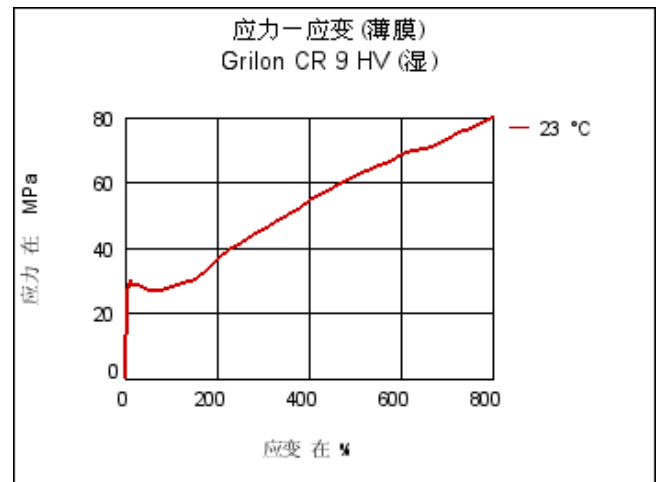
应力 - 应变(薄膜)
